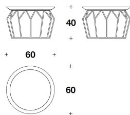
TCV (19) LOW : SIDE TABLE Ø 60x40H.cm Ø 23 2/3x15 3/4H."
