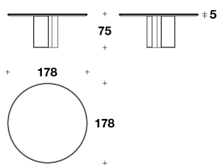
LLT (24E) - LLT (24V) TAVOLO TONDO / ROUND TABLE Ø 178x75H. - THK.5 cm Ø 70x29 2/3H. - THK.1 15/16 "
