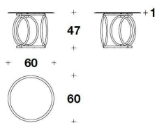
CTT (23V) - CTT (23M) SIDE TABLE Ø 60x47H.cm Ø 23 2/3x18 2/4H."
