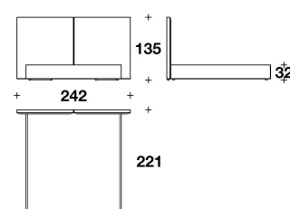
LFD (KUSA) KING USA : LETTO PER MATERASSO / BED FOR MATTRESS 195x205 - 242x221x135H. - H.B.32cm 76 2/3x80 2/3 - 95 1/3x87x53H. - H.B.12 2/4"
