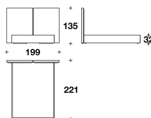
LFD (QUSA) QUEEN USA : LETTO PER MATERASSO / BED FOR MATTRESS 152x205 - 199x221x135H. - H.B.32cm 60x80 2/3 - 78 1/3x87x53H. - H.B.12 2/4"
