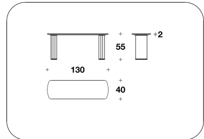
CTB (28PE) - CTB (28PP) - CTB (28VE) - CTB (28VP) SIDE TABLE 130x40x55H.cm 51 1/3x15 3/4x21 2/3H."
