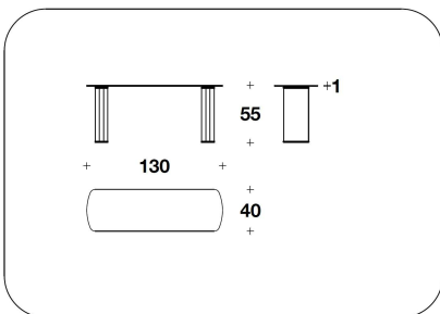
CTB (28PE) - CTB (28PP) - CTB (28VE) - CTB (28VP) SIDE TABLE 130x40x55H.cm 51 1/3x15 3/4x21 2/3H."
