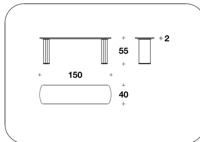
CTB (26PE) - CTB (26PP) - CTB (26VE) - CTB (26VP) SIDE TABLE 150x40x55H.cm 59x15 3/4x21 2/3H."
