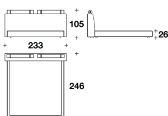
ELN (KUSA) KING USA : LETTO PER MATERASSO / BED FOR MATTRESS 195x205 - 233x246x105H. - H.B.26cm 76 2/3x80 2/3 - 91 2/3x97x41 1/3H. - H.B.10 1/4"
