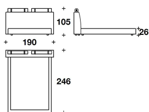
ELN (QUSA) QUEEN USA : LETTO PER MATERASSO / BED FOR MATTRESS 152x205 - 190x246x105H. - H.B.26cm 60x80 2/3 - 74 2/3x97x41 1/3H. - H.B.10 1/4"
