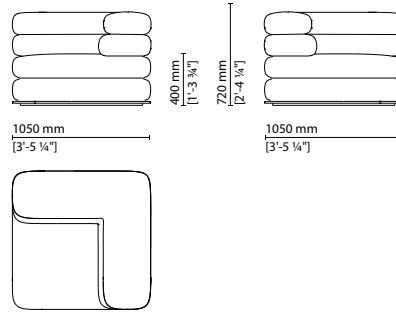
078 019 — Left corner element
