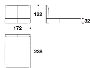
EDM (QUSA) QUEEN USA : LETTO PER MATERASSO / BED FOR MATTRESS 152x205 - 172x238x122H. - H.B.32cm 60x80 2/3 - 67 2/3x93 2/3x48H. - H.B.12 2/4"
