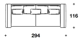
ELN (AE1D) + ELN (AE1S) A) : ESEMPIO DI COMPOSIZIONE / SECTIONAL SOFA EXAMPLE 294x116x98H. - H.S.47 cm 115 2/3x45 2/3x38 2/3H. - H.S.18 2/4 "
