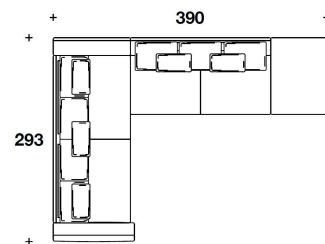
ELN (AD4AS) + ELN (AE2C) + ELN (POUR) D) : ESEMPIO DI COMPOSIZIONE / SECTIONAL SOFA EXAMPLE 390x293x98H. - H.S.47 cm 153 1/2x115 1/3x38 2/3H. - H.S.18 2/4 "
