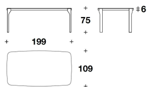
TTV (20MF) - TTV (20PF) TAVOLO / TABLE 199x109x75H. - THK.6cm 78 1/3x43x29 2/3H. - THK.2 6/16"
