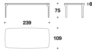
TTV (21MF) - TTV (21PF) TAVOLO / TABLE 239x109x75H. - THK.6cm 94x43x29 2/3H. - THK.2 6/16"
